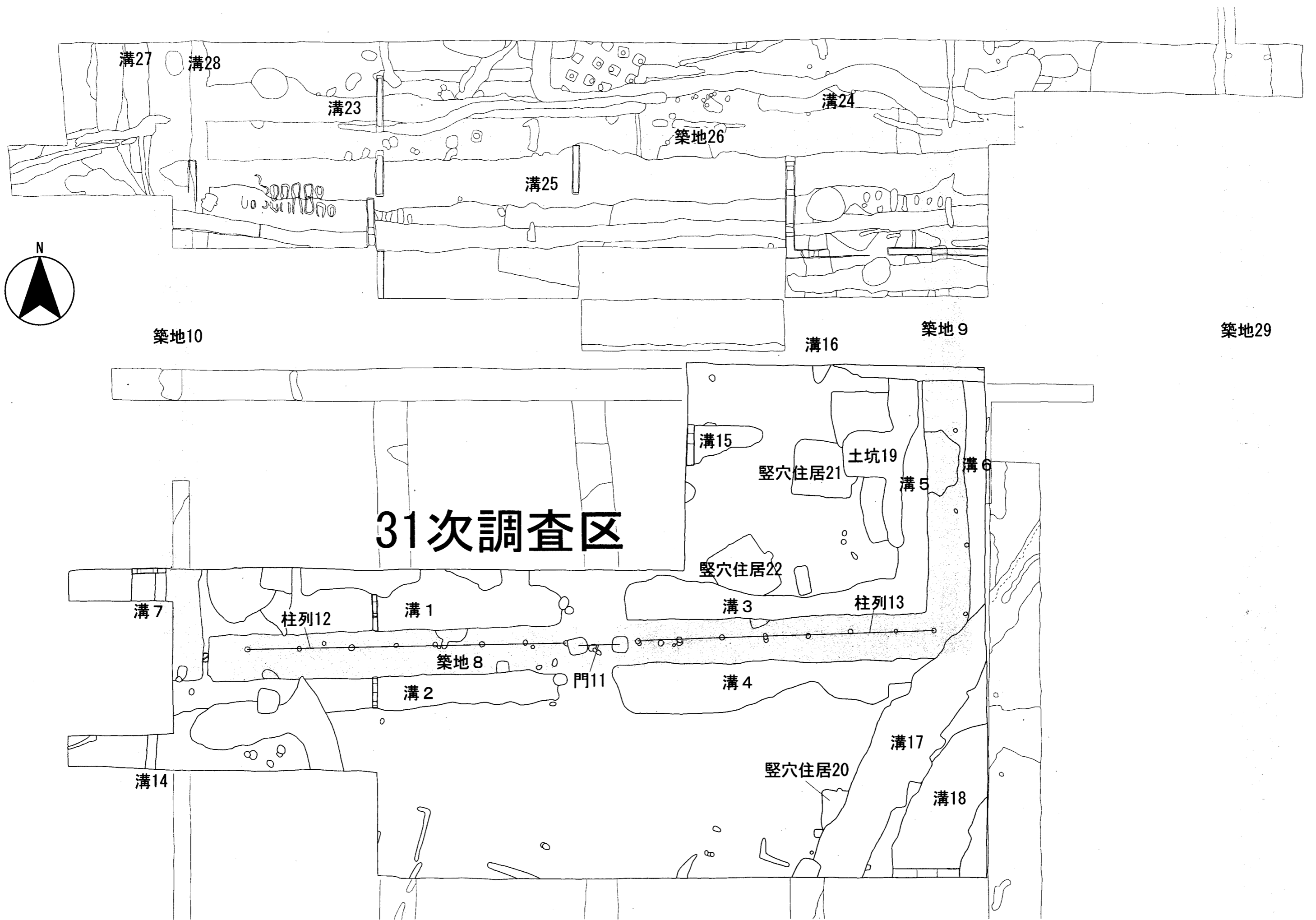
遺構位置図・院推定復元図 (1 : 200)
